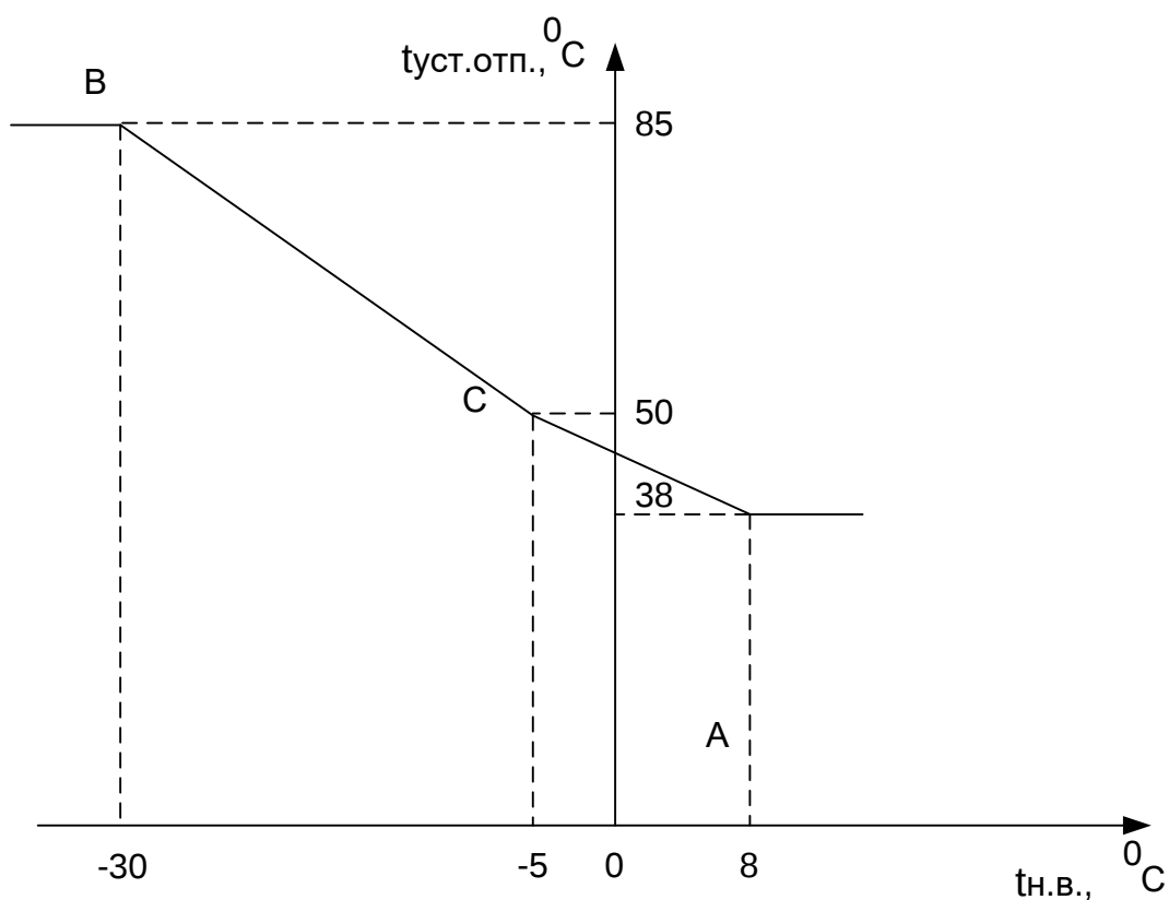
Рисунок П8.1 Зависимость установки температуры отопления от температуры подающего трубопровода t_{уст.отп.} = f(t_{н.в.})
