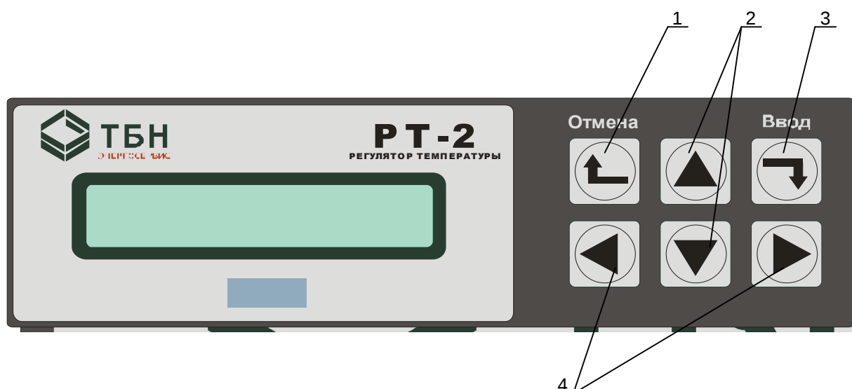
Рисунок 4 Лицевая панель РТ-2М
