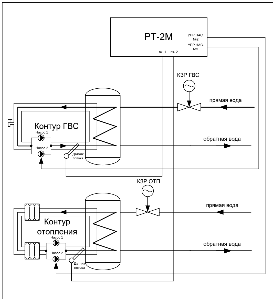
Рисунок П 2.1 Схема подключения регулятора РТ-2М при использовании на ЦТП (ИТП) для управления работой насосов.
