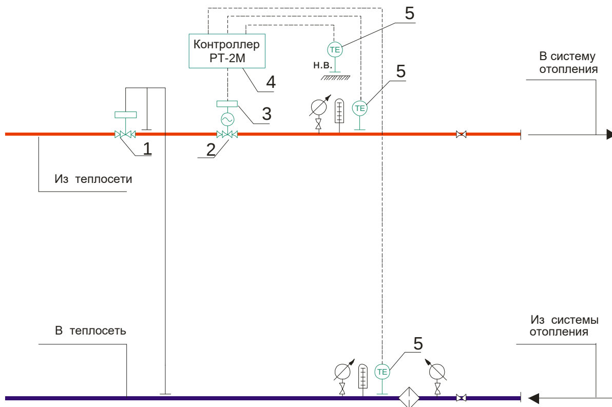
Рисунок ПЗ.4 Принципиальная гидравлическая схема узла регулирования для системы ОТП.
