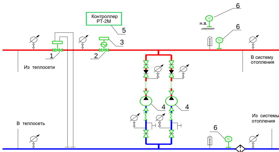
Рисунок ПЗ.1 Принципиальная гидравлическая схема подключения с насосами на перемычке.
