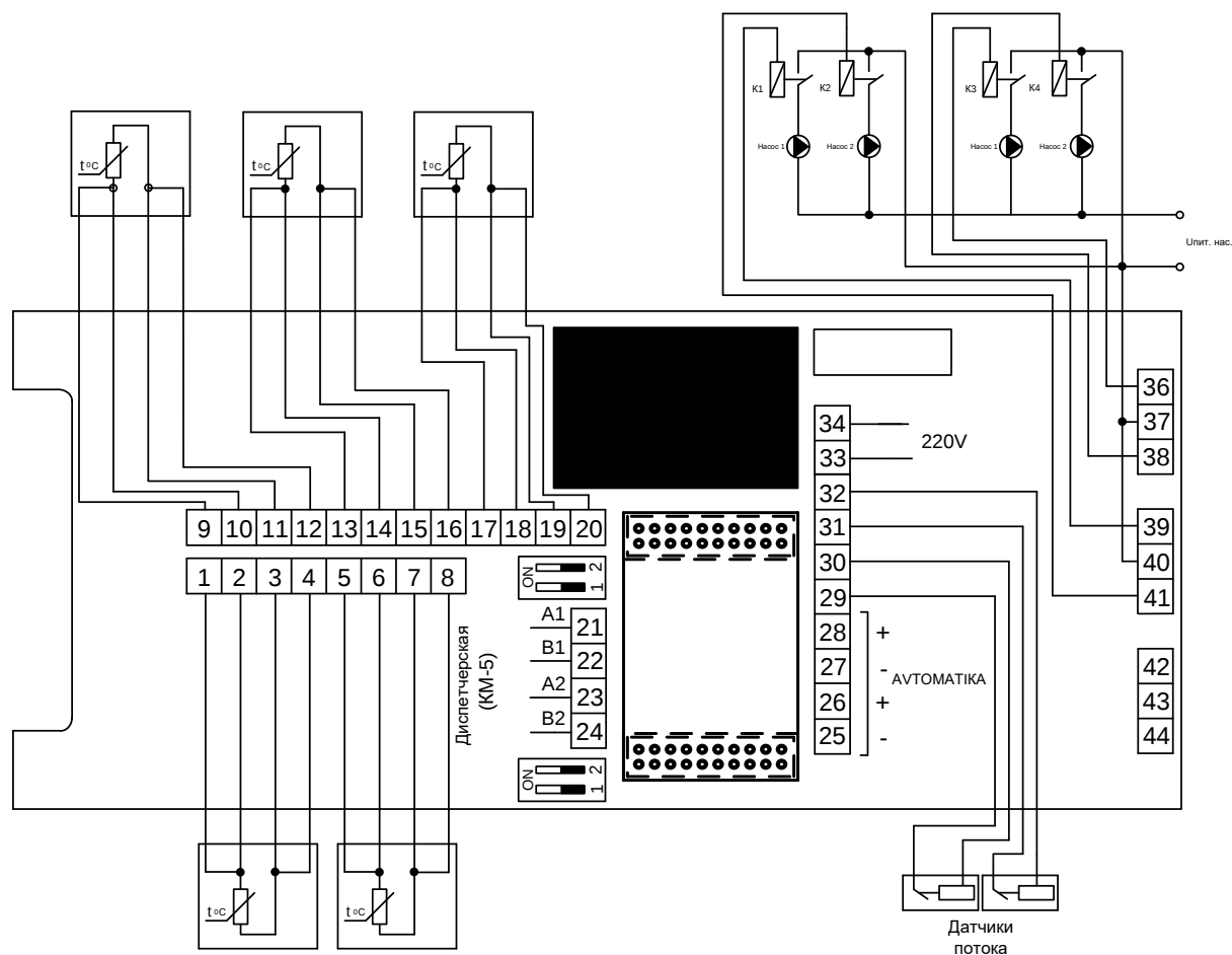
Рисунок П 1. 2 Схема подключения насосов и датчиков потока.
