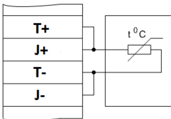
Рисунок П4.2 Двухпроводная схема подключения термометров-сопротивлений
