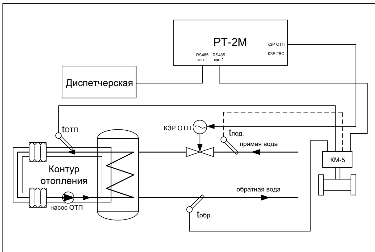
Рисунок П 2.2 Схема подключения регулятора РТ-2М на узле регулирования и учета при совместном использовании с теплосчетчиком КМ-5 .
