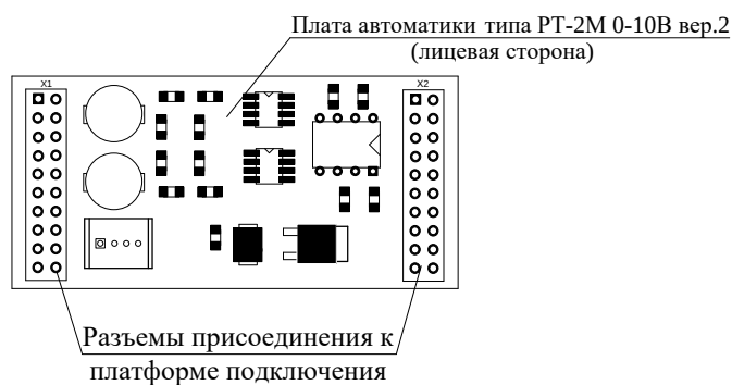
Рисунок 2 Плата автоматики
