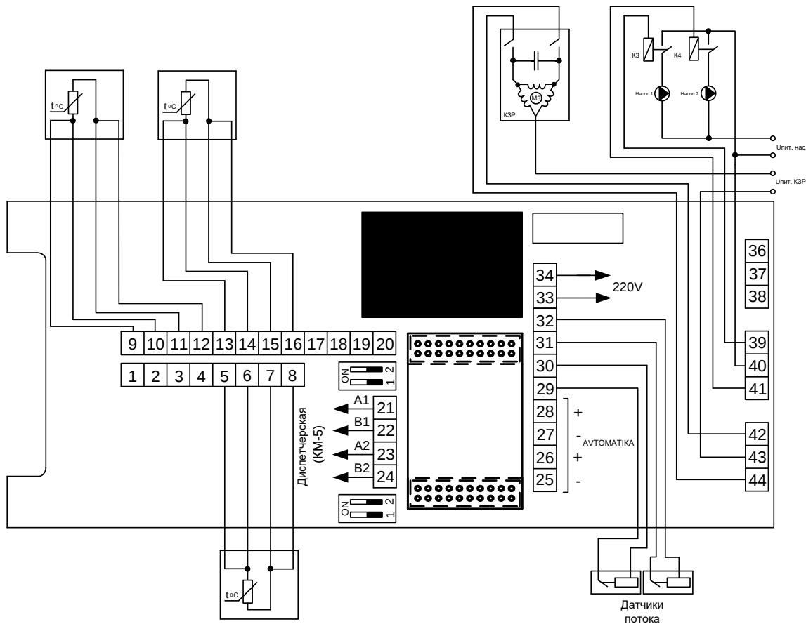
Рисунок ПЗ. 3 Электрическая схема подключения (для гидравлических схем, приведенных на Рисунок ПЗ.1 и Рисунок ПЗ. 2)
