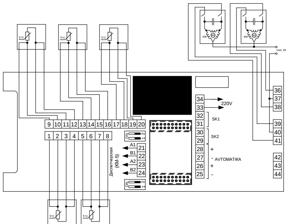
Рисунок П 1.1 Схема электрических подключений РТ-2М при использовании в качестве исполнительных механизмов КЗР с дискретным управлением.
