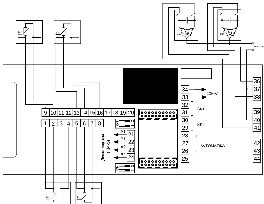
Рисунок ПЗ. 7 Электрическая схема подключения (для схемы подключения регулятора РТ-2М, приведенной на Рисунок ПЗ. 6 ).
