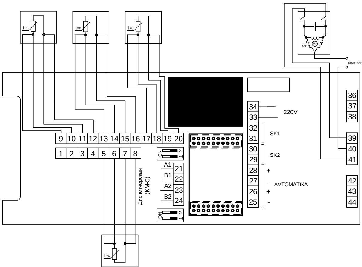
Рисунок ПЗ.5 Электрическая схема подключения (для гидравлической схемы, приведенной на Рисунок ПЗ.4).
