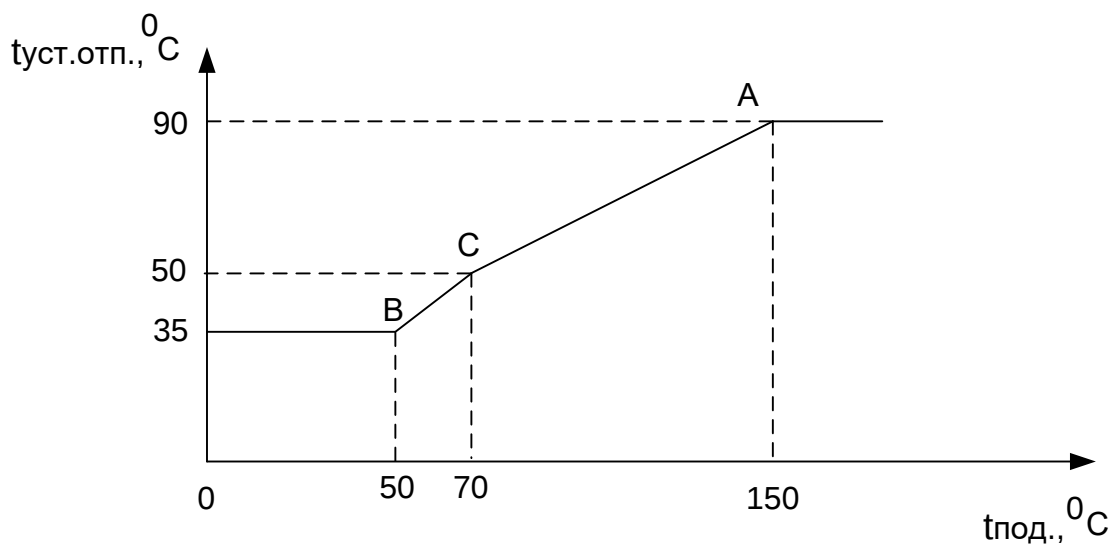
Рисунок П8.2 Зависимость установки температуры отопления от температуры подающего трубопровода t_{уст.отп.} = f(t_{под.})
