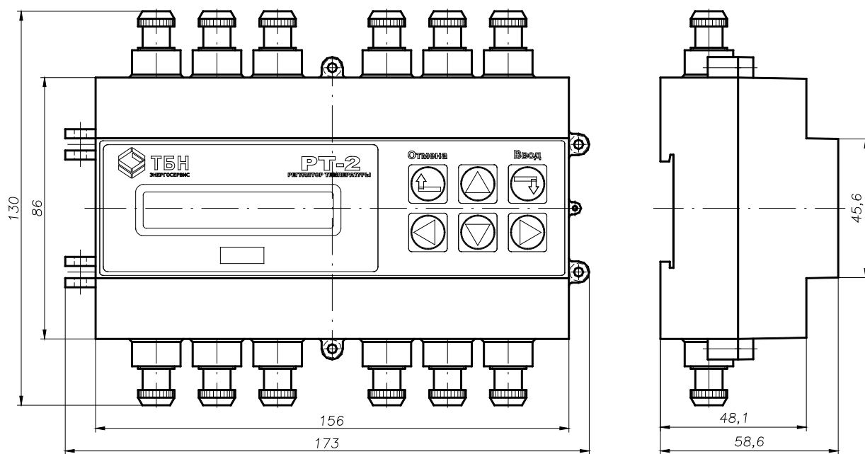
Рисунок 3 Внешний вид РТ-2М.
