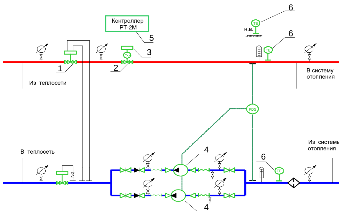
Рисунок ПЗ. 2 Принципиальная гидравлическая схема подключения с насосами на обратном трубопроводе.
