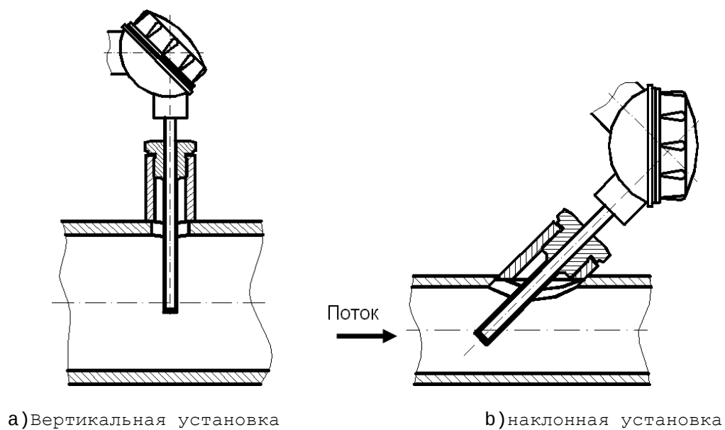
Рисунок П4.1 Вертикальная и наклонная установка термометров.
