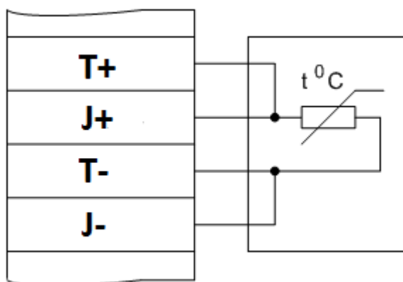
Рисунок П4.3 Четырехпроводная схема подключения термометров-сопротивлений
