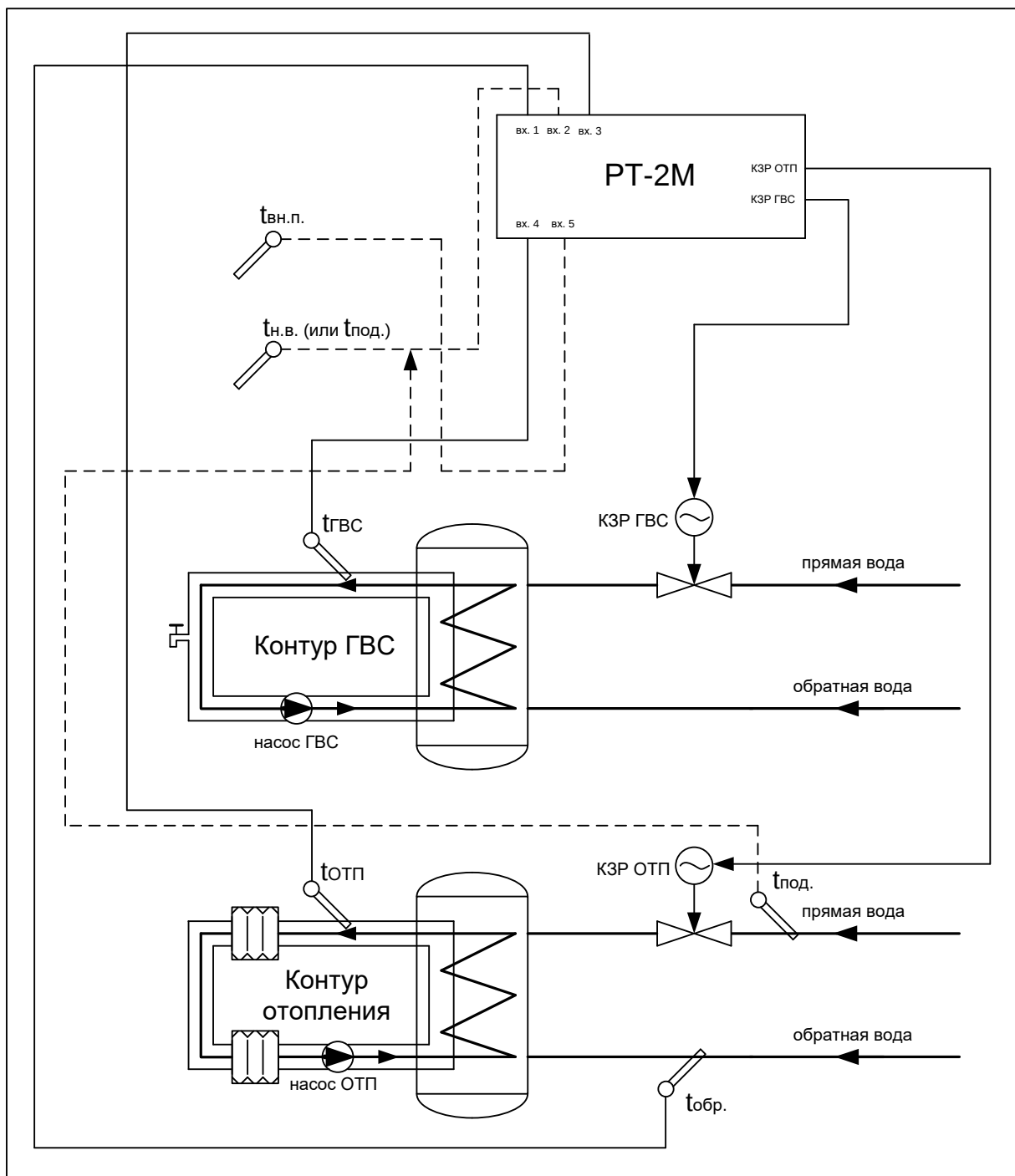
Рисунок ПЗ. 6 Схема подключения регулятора РТ-2М при использовании на ЦТП (ИТП) для регулирования системы ОТП и системы ГВС.
