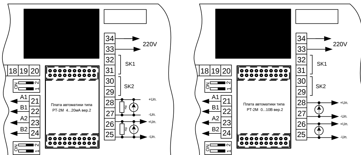
Рисунок П 1. 3 Схема подключения исполнительных механизмов с управлением напряжением 0...10В и током 4...20мА к выходам ЦАП регулятора РТ-2М.
