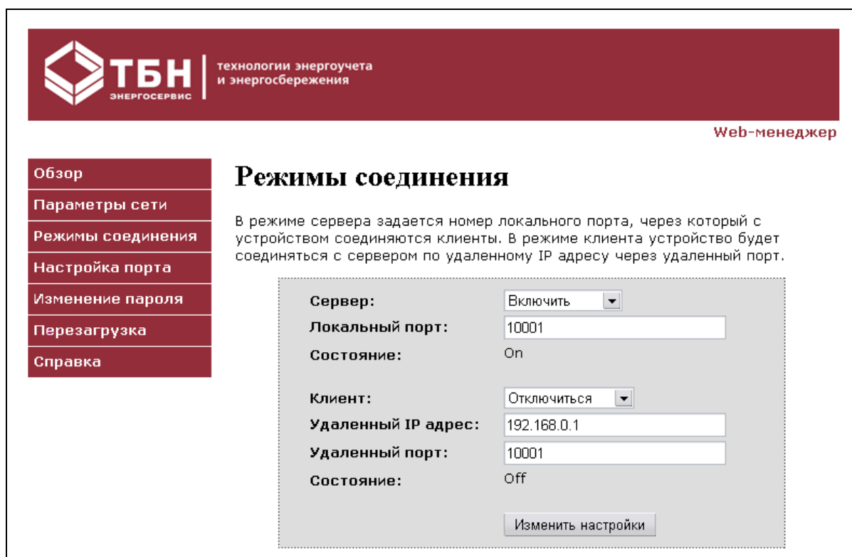
Рисунок ПЗ.14. Окно пункта «WEB-страница» страница Режимы соединения
