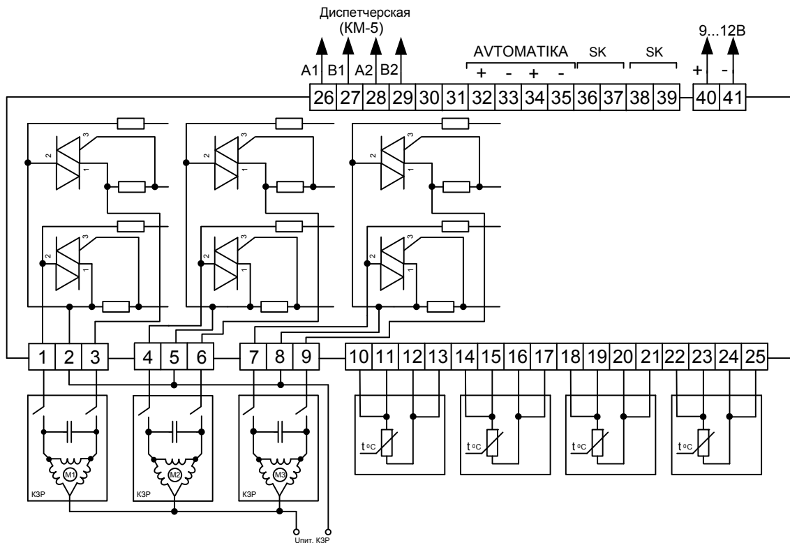
Рисунок П 1.1. Схема электрических подключений РТ-2 при использовании в качестве исполнительных механизмов КЗР с дискретным управлением.
