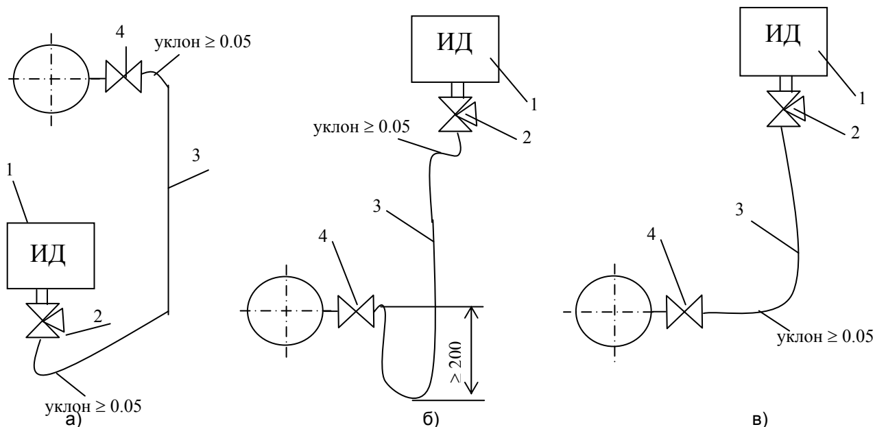
Рисунок 2 — Установка датчика для измерения давления неагрессивной жидкости и пара до P_y \leq 1,6 МПа и при температуре до 100\text{ }^\circ\text{C}
