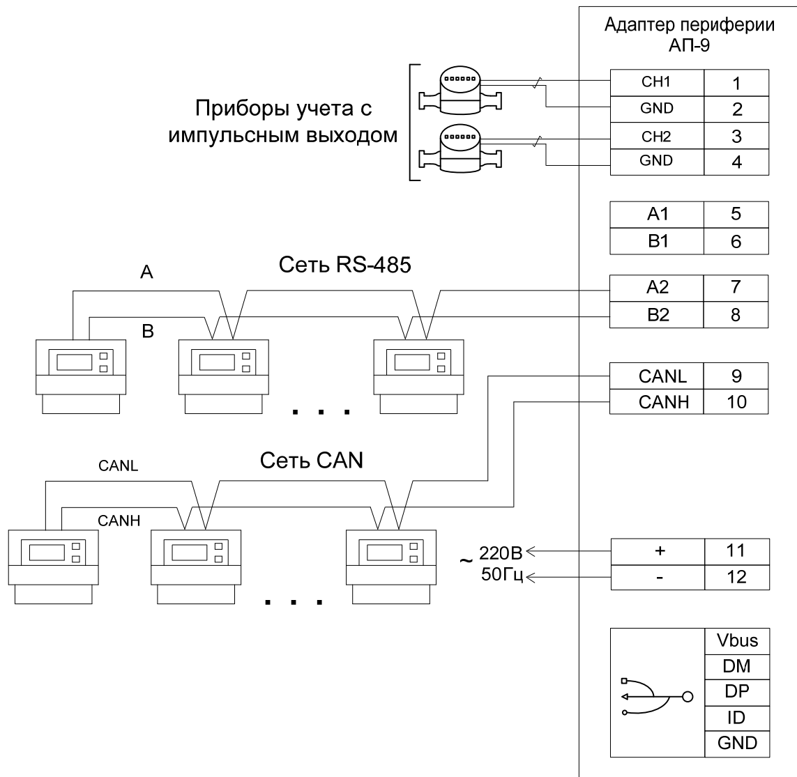
Рисунок П 2.1 Монтаж электрических цепей для модификации АП-9-2И
